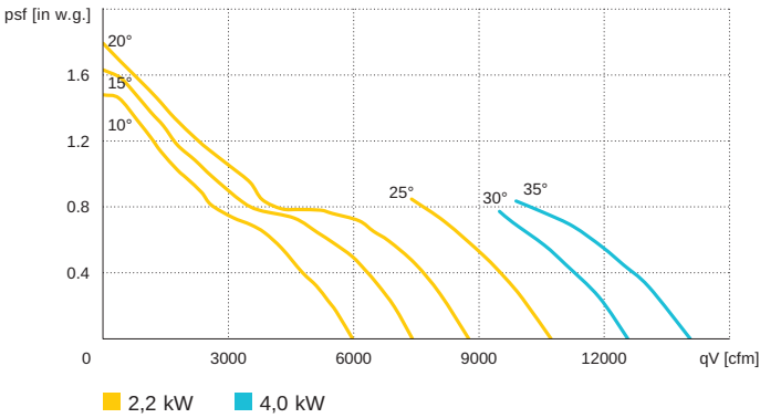
AL 710 D6 / 50 Hz
