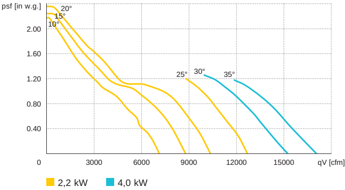
AL 800 D6 / 60 Hz
