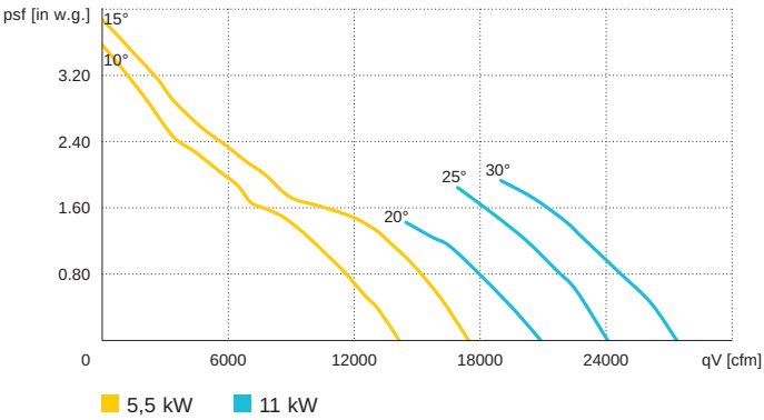
AL 900 D6 / 60 Hz
