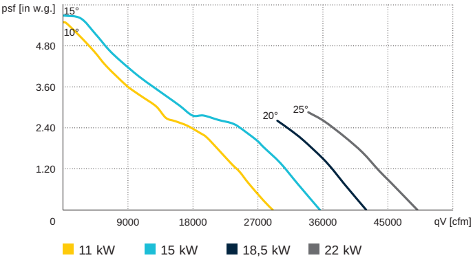
AL 1120 D6 / 60 Hz
