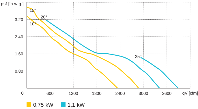
AL 400 D2 / 50 Hz
