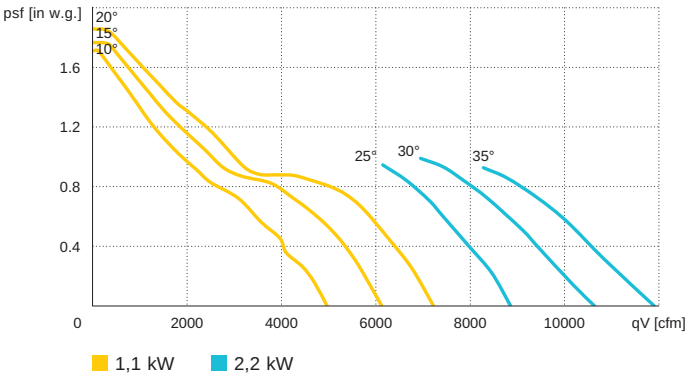
AL 710 D6 / 60 Hz
