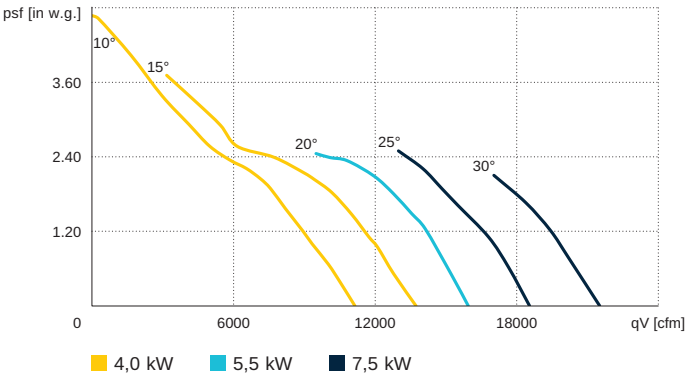
AL 800 D4 / 60 Hz
