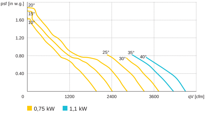
AL 500 D4 / 60 Hz
