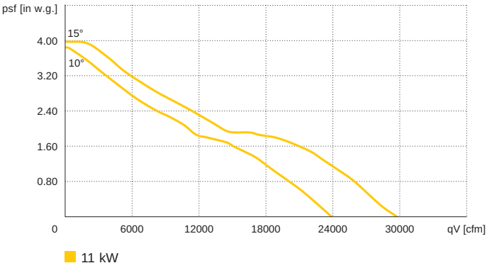
AL 1120 D6 / 50 Hz
