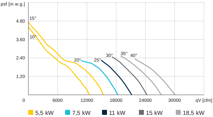
AL 800 D4 / 50 Hz
