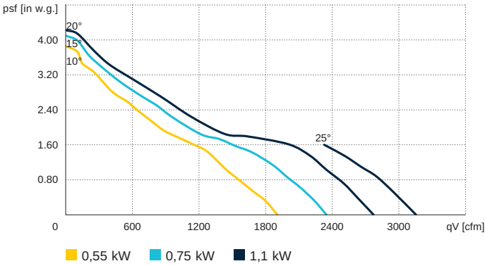
AL 355 D2 / 60 Hz
