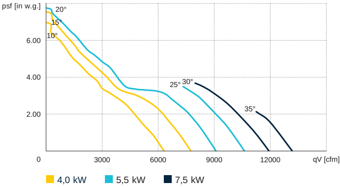
AL 560 D4 / 50 Hz
