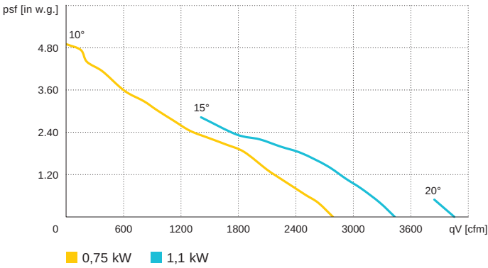
AL 400 D2 / 60 Hz
