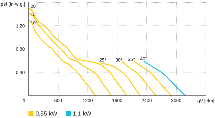
AL 400 D4 / 60 Hz
