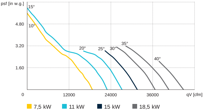
AL 1000 D4 / 50 Hz
