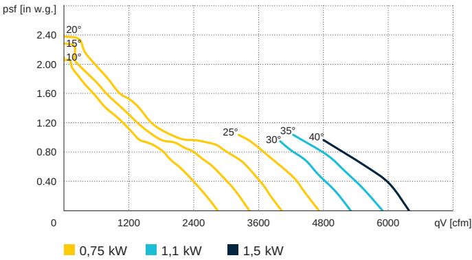
AL 450 D4 / 60 Hz
