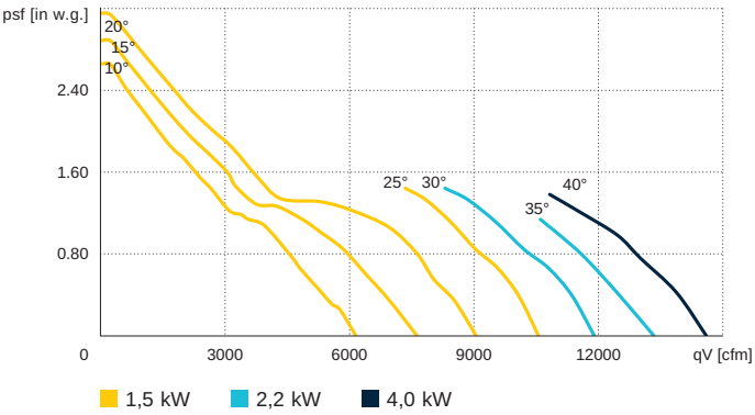
AL 710 D4 / 50 Hz
