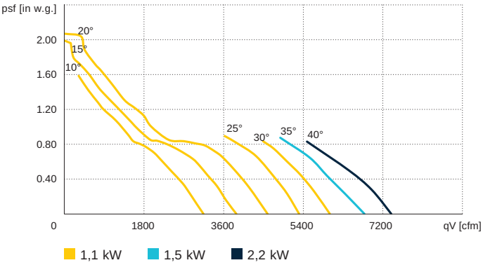
AL 630 D4 / 50 Hz
