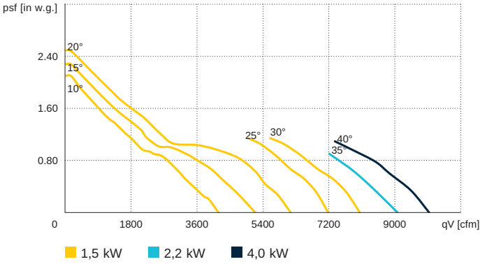
AL 630 D6 / 50 Hz
