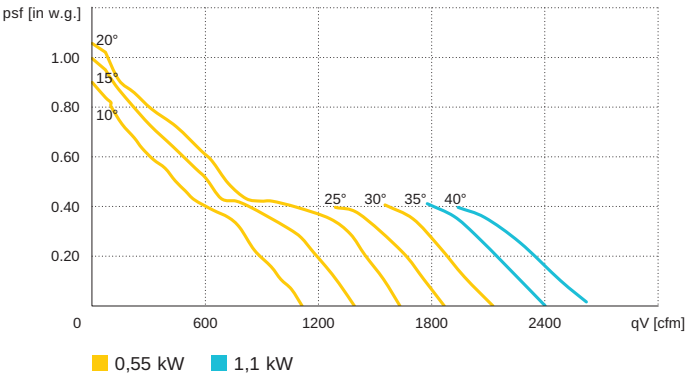
AL 400 D4 / 50 Hz
