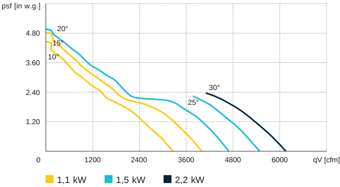
AL 450 D2 / 50 Hz
