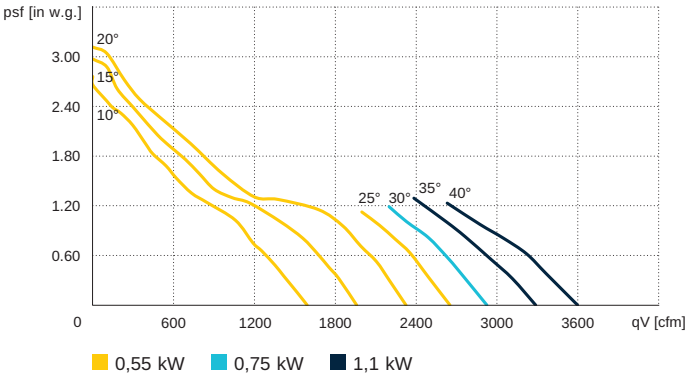
AL 355 D2 / 50 Hz
