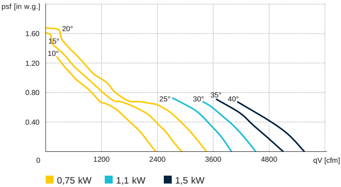
AL 450 D4 / 50 Hz
