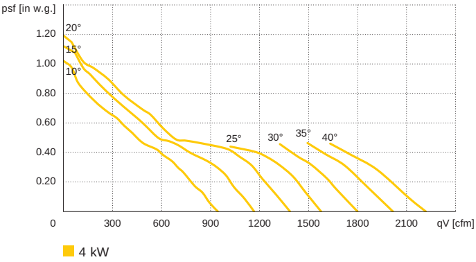
AL 355 D4 / 60 Hz
