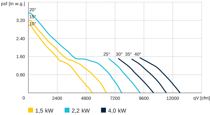
AL 630 D6 / 60 Hz
