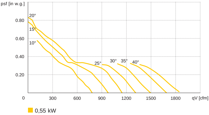
AL 355 D4 / 50 Hz
