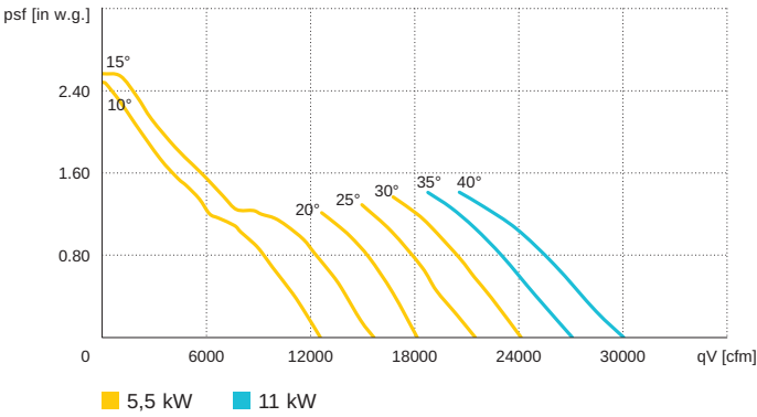
AL 1000 D6 / 50 Hz
