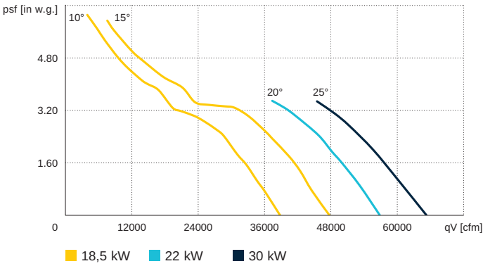
AL 1250 D6 / 60 Hz
