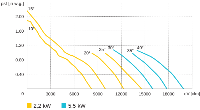
AL 900 D6 / 50 Hz
