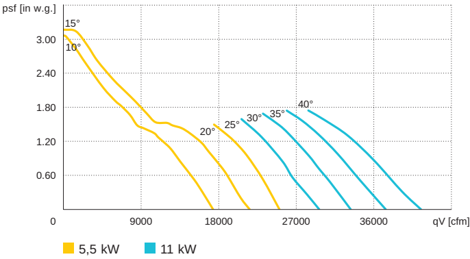
AL 1250 D6 / 50 Hz
