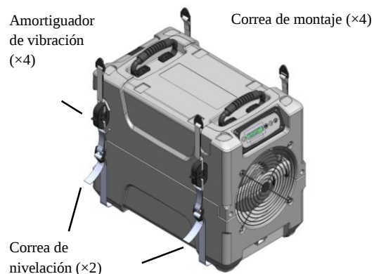
Fig. B: Correas de suspensión
