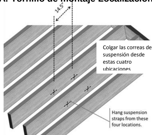
Fig. A: Tornillo de montaje Localización
