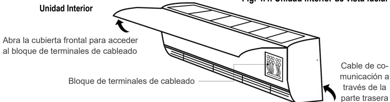
Fig. 4.4: Unidad interior de vista facial
