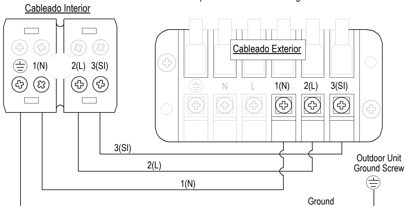
Fig. 4.4b: Diagrama de cableado
