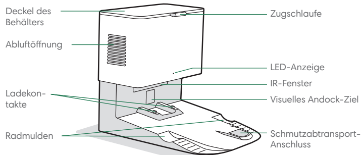
Vorderansicht
