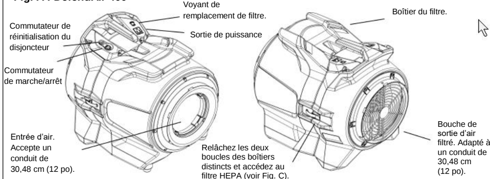
Fig. A : DefendAir 400
