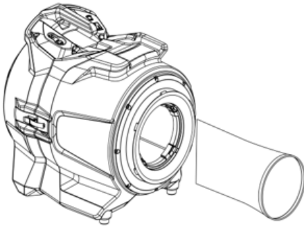
Fig. B : Remplacement du préfiltre
