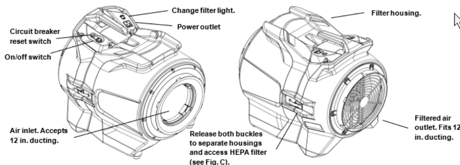
Fig. A: DefendAir 400
