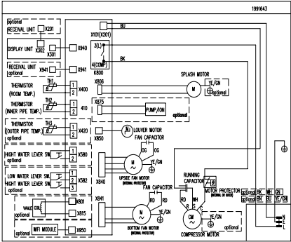
Esquema eléctrico
