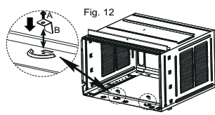
A. Tornillos Philips cabeza plana de 10 x 1/2" B. Tornillos cabeza redonda de 10 x 3/4" C. Canal de ventana
