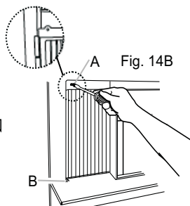
A. Tornillos cabeza redonda de 10 x 3/4" (o 1/2") B. Orificio ranurado en la parte inferior de la cortina
