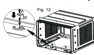
A. Tornillos Philips cabeza plana de 10 x 1/2" B. Tornillos cabeza redonda de 10 x 3/4" C. Canal de ventana
