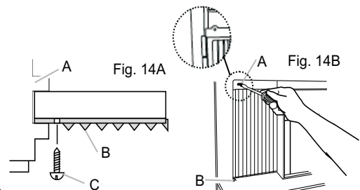
A. Canal de ventana B. Cortina izquierda C. Tornillos cabeza redonda de 10 x 3/4" (o 1/2")
