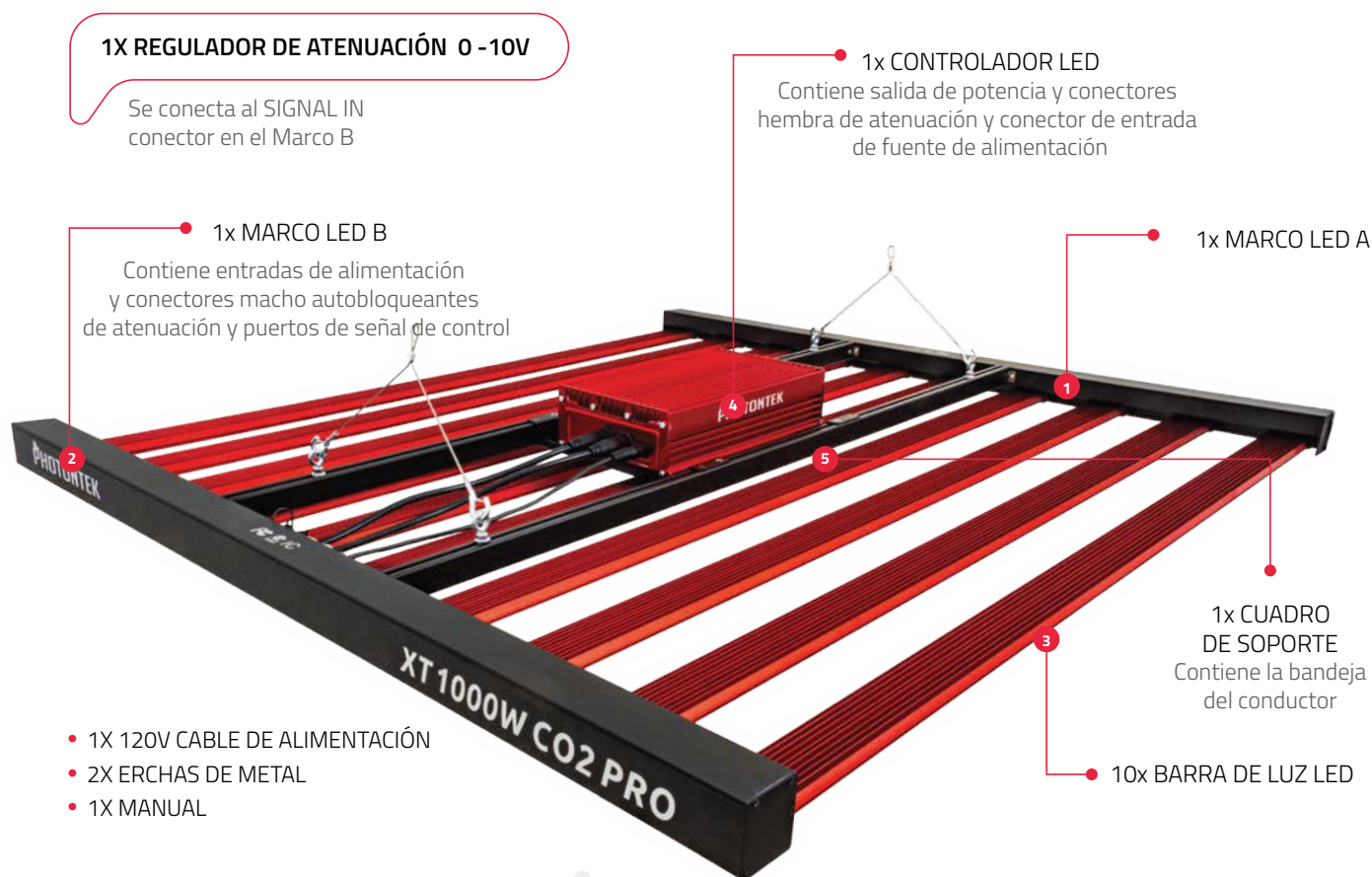
Fig4. Componentes del accesorio.
