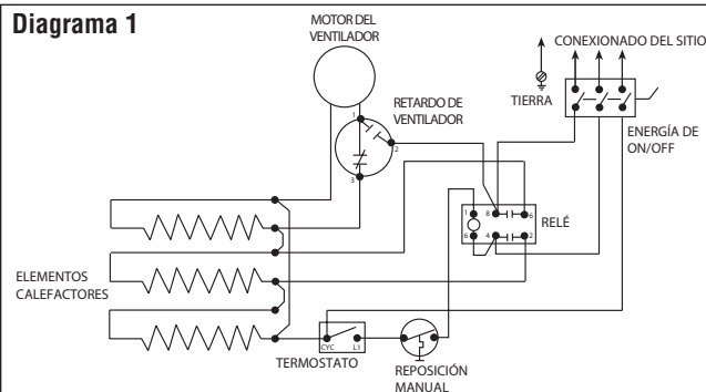
DIAGRAMA DE CONEXIONADO PARA CALEFACTORES DE PARED TRIFÁSICOS
