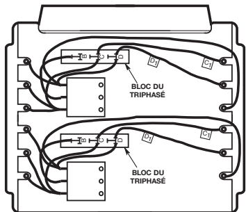
CÂBLAGE D'USINE POUR ALIMENTATION EN MONOPHASE
