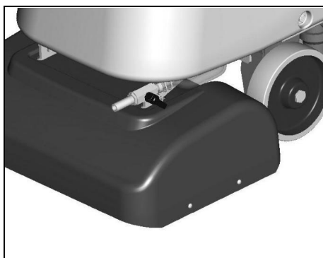
Dispositif de vidange de la solution détergente
