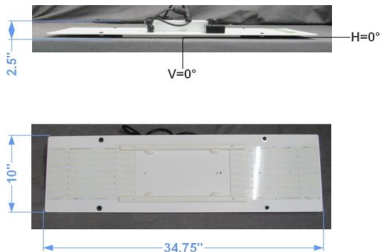
FIG. 1 LUMINAIRE
