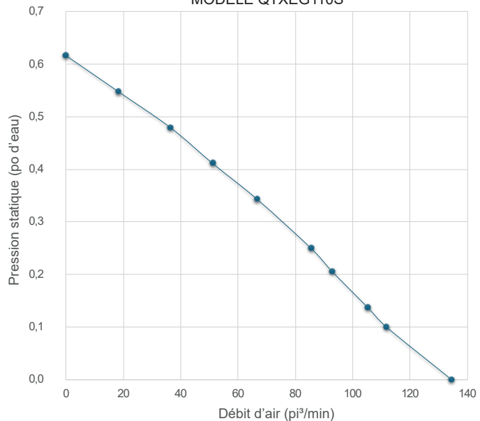
MODÈLE QTXEG110S
