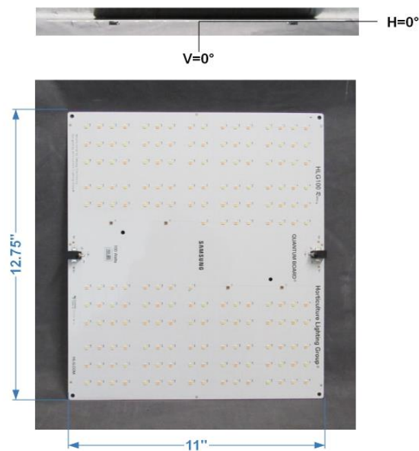
FIG. 1 LUMINAIRE
