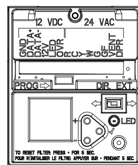
ÉCRAN ET CONNEXIONS BAS VOLTAGE
